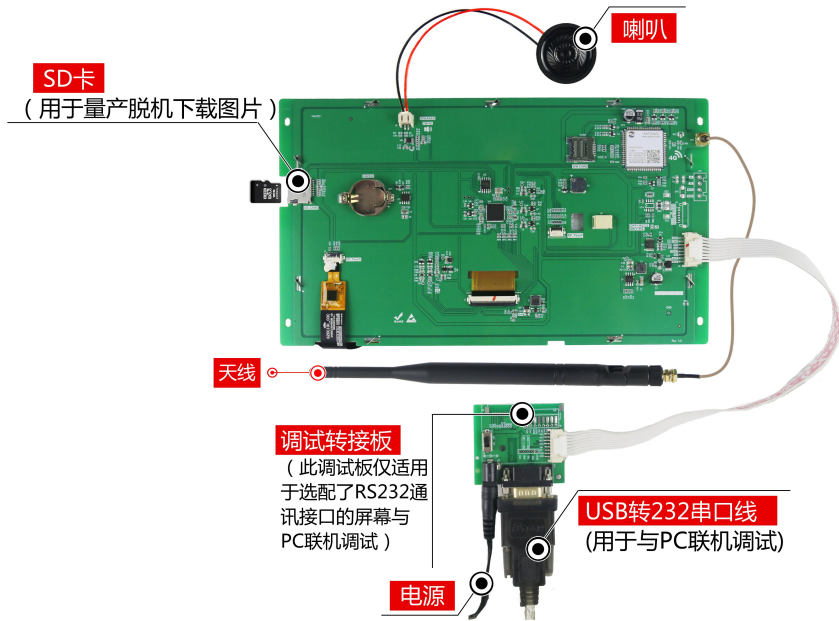
图 1-5 调试工具图
