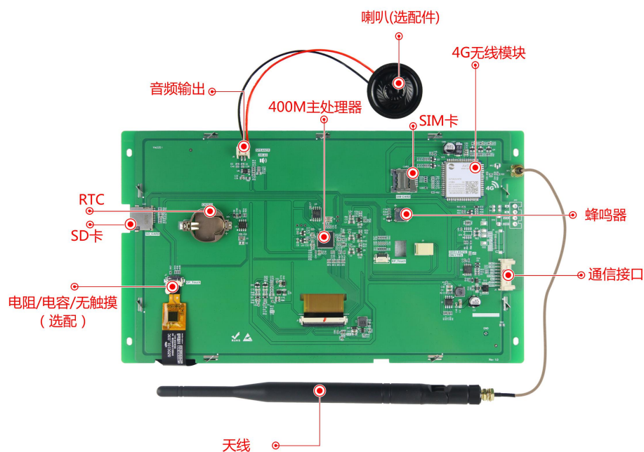
图 1-4 硬件配置图
